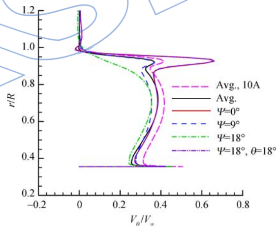
(b) 周向速度沿径向的分布
