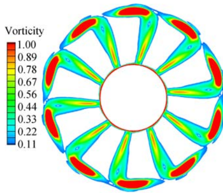
(a) 前转子后 0.2R 流向位置处涡量分布
