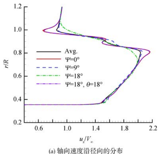
(a) 轴向速度沿径向的分布
