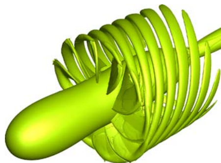
(a) 单个转子
