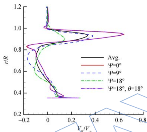
(b) 周向速度沿径向的分布
