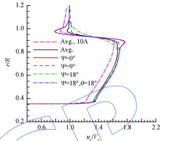
(a) 轴向速度沿径向的分布
